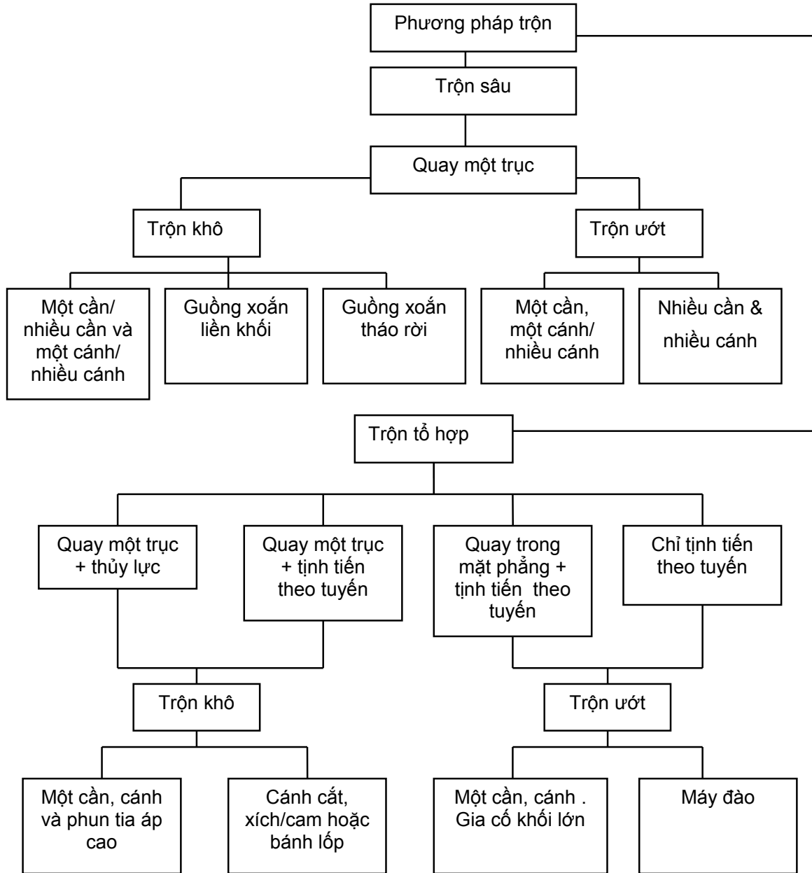
Hình A.1 - Phân loại chung các thiết bị trộn trộn sâu
