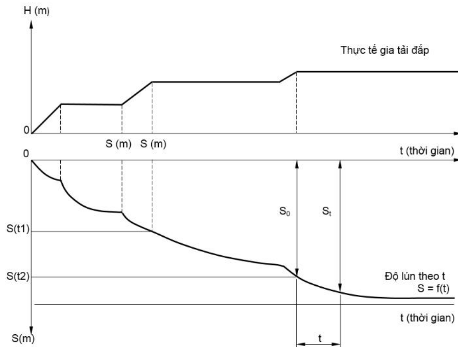
Hình D.1 – Đồ thị quan trắc lún và diễn biến thực tế gia tải đắp theo thời gian
