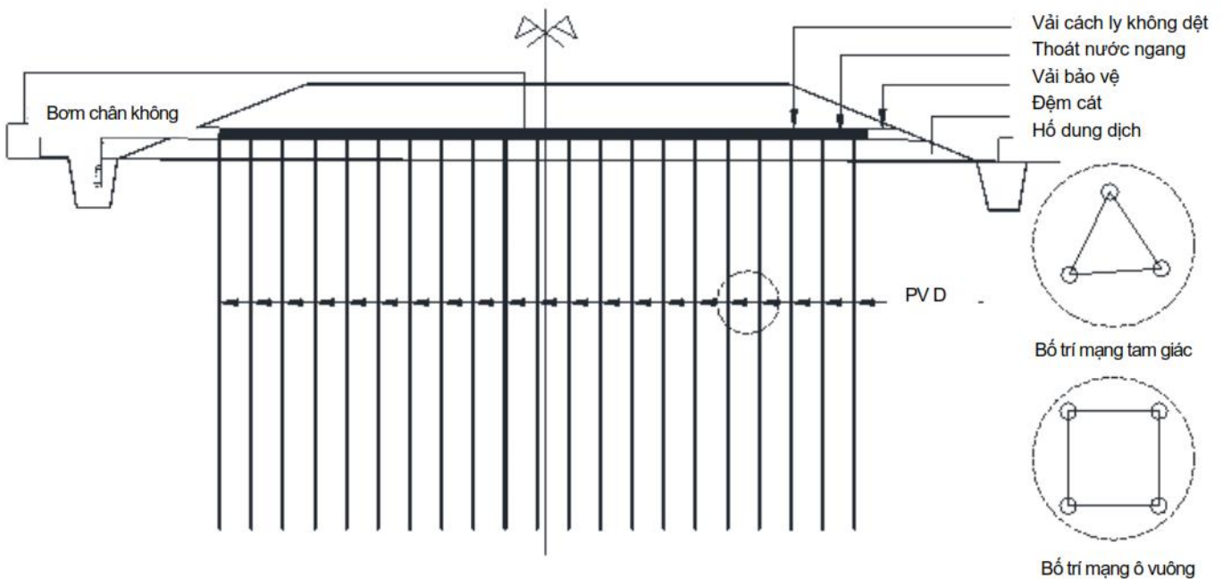
Hình E.4 – Xử lý đất yếu bằng công nghệ bấc thấm kết hợp cố kết chân không.
